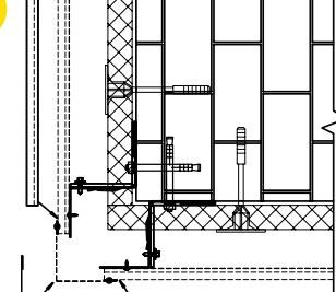
Внешний угол здания. Горизонтальный разрез. Простой угол.
